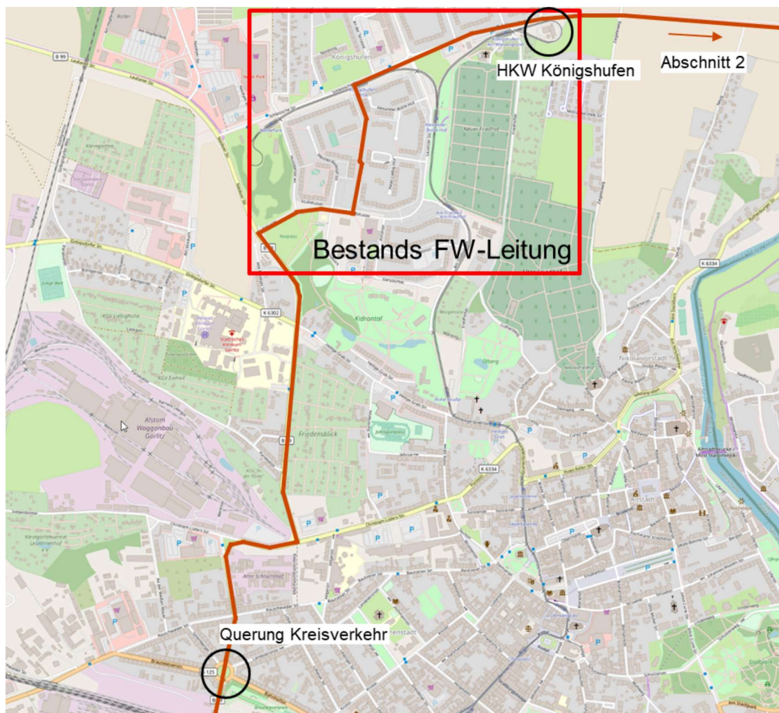
Abbildung 23: Geplanter Trassenverlauf und kritische Stellen der Verbindung Königshufen bis Brautwiesenstraße.
